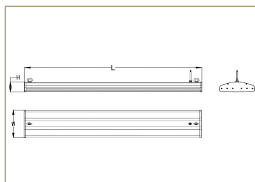
Dimensions : modèle PROXI-ARENA-L
