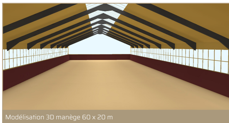
Simulation Dialux 36 luminaires (Éclairage moyen 407 lx - Uniformité 0,73)
